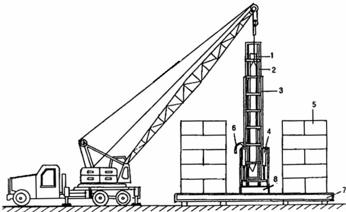
Hình A2.1 Máy ép đỉnh: 1 - Cọc ép; 2 - Khung dẫn hướng di động; 3 - Khung dẫn hướng cố định; 4 - Xi lanh ép; 5 - Đồi trọng (tải); 6 - Ống mềm dẫn dầu thủy lực; 7 - Khung chính; 8 - Khung phụ
