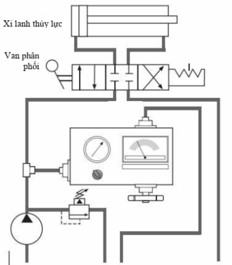
Hình B4 Sơ đồ lắp bộ thiết bị kiểm tra hoạt động và độ kín trong của xi lanh thủy lực và van van phân phối
