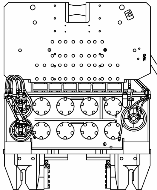
Hình A1.4.2 Máy đóng cọc bánh xích
