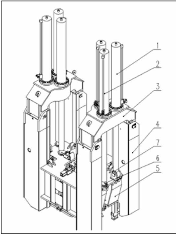
Hình A2.2.2 Cấu tạo của cơ cấu ép cọc: 1, 2 - Các xi lanh thủy lực ép cọc (chính và phụ); 3 - Dầm ngang đỡ các xi lanh thủy lực ép cọc; 4 - Trụ đỡ dẫn hướng ép cọc; 5 - Hộp kẹp cọc; 6 - Ấc và chốt ghép cần của xi lanh thủy lực ép cọc với hộp kẹp cọc; 7 - Bát cầu trên hộp kẹp cọc 5 có nhiệm vụ tiếp nhận đầu dạng cầu tròn của các xi lanh thủy lực ép cọc phụ
