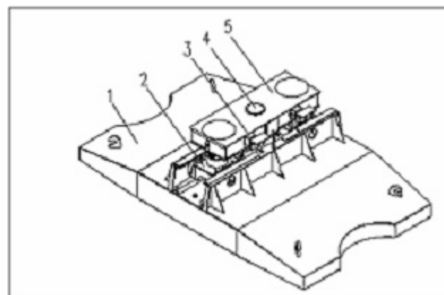
Hình A2.2.6 Cấu tạo cơ cấu di chuyển ngang và quay: 1 - Chân di chuyển ngang; 2 - Cụm bánh sắt di chuyển ngang; 3 - Lò xo; 4 - Ổ trục quay trung tâm; 5 - Bàn quay.
